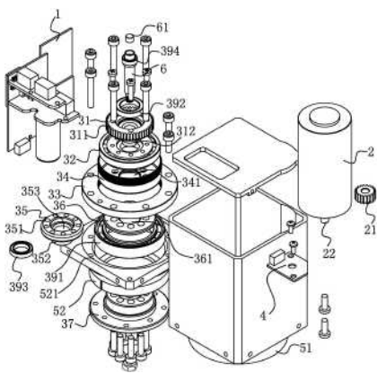
图示：优必选伺服电机专利 一种伺服电机及其控制方法 CN106208543B
